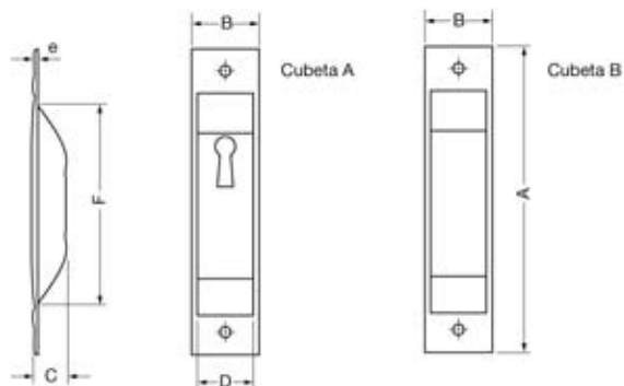
Cuadro de medidas (mm.)
